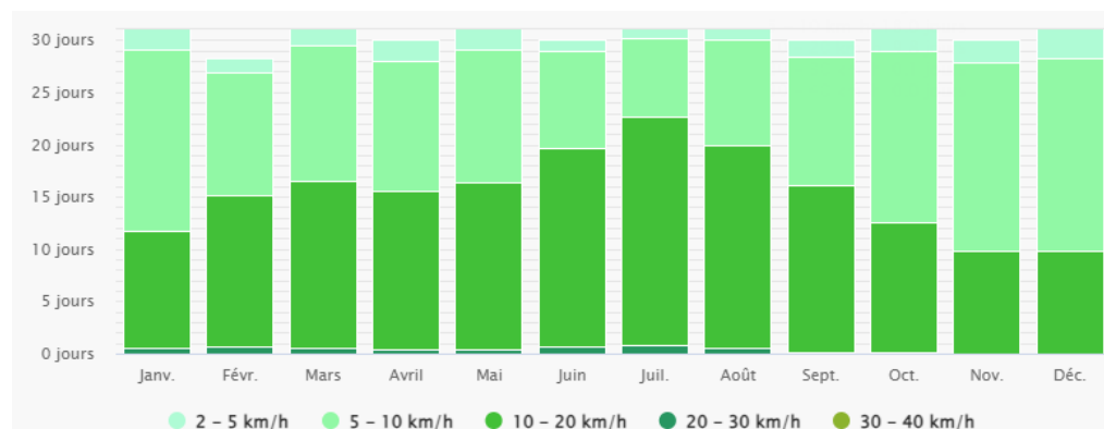
Figure 1 : Vitesses de vents moyennes mensuelles
