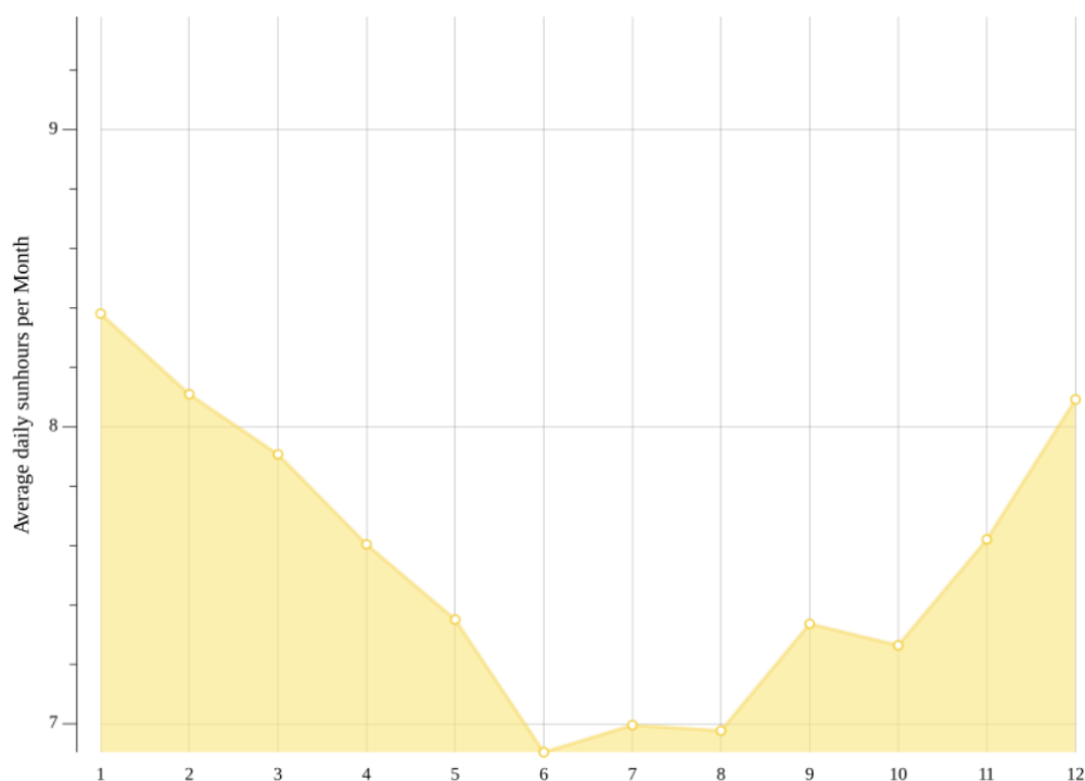
Figure 2 : Durée moyenne d'ensoleillement quotidien par mois (Climate Data, 2021)
